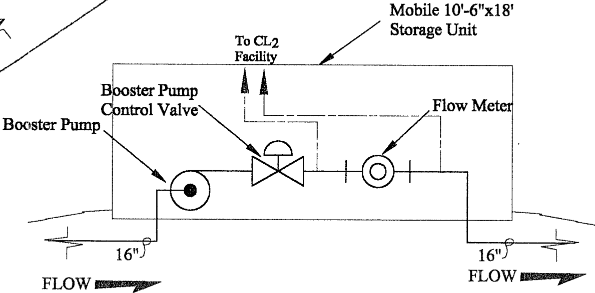
Detail A-A' Scale: NTS
